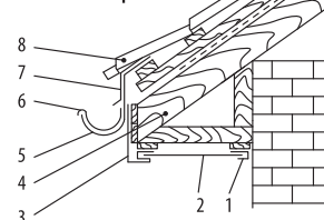
Рис. 3.8 Карниз
